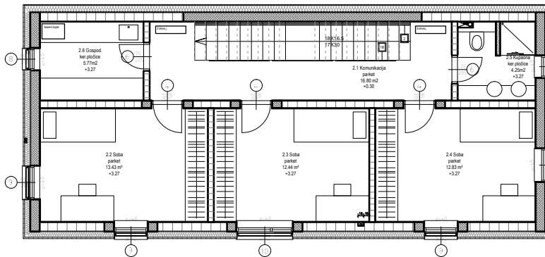
TLOCRT 1. KATA
