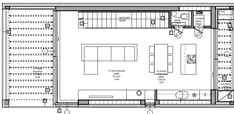
TLOCRT 2. KATA
