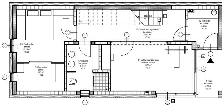
TLOCRT PRIZEMLJA
